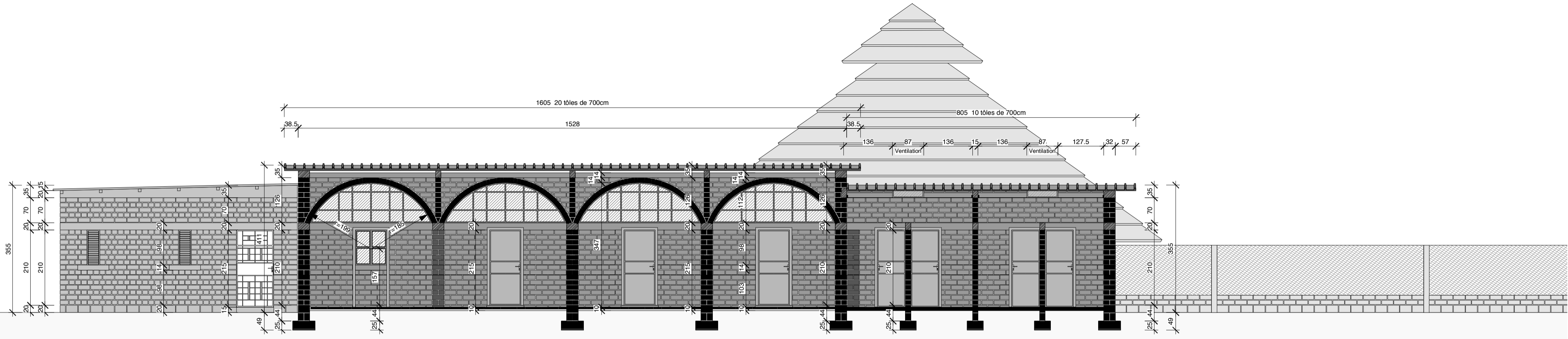
COUPE KK
